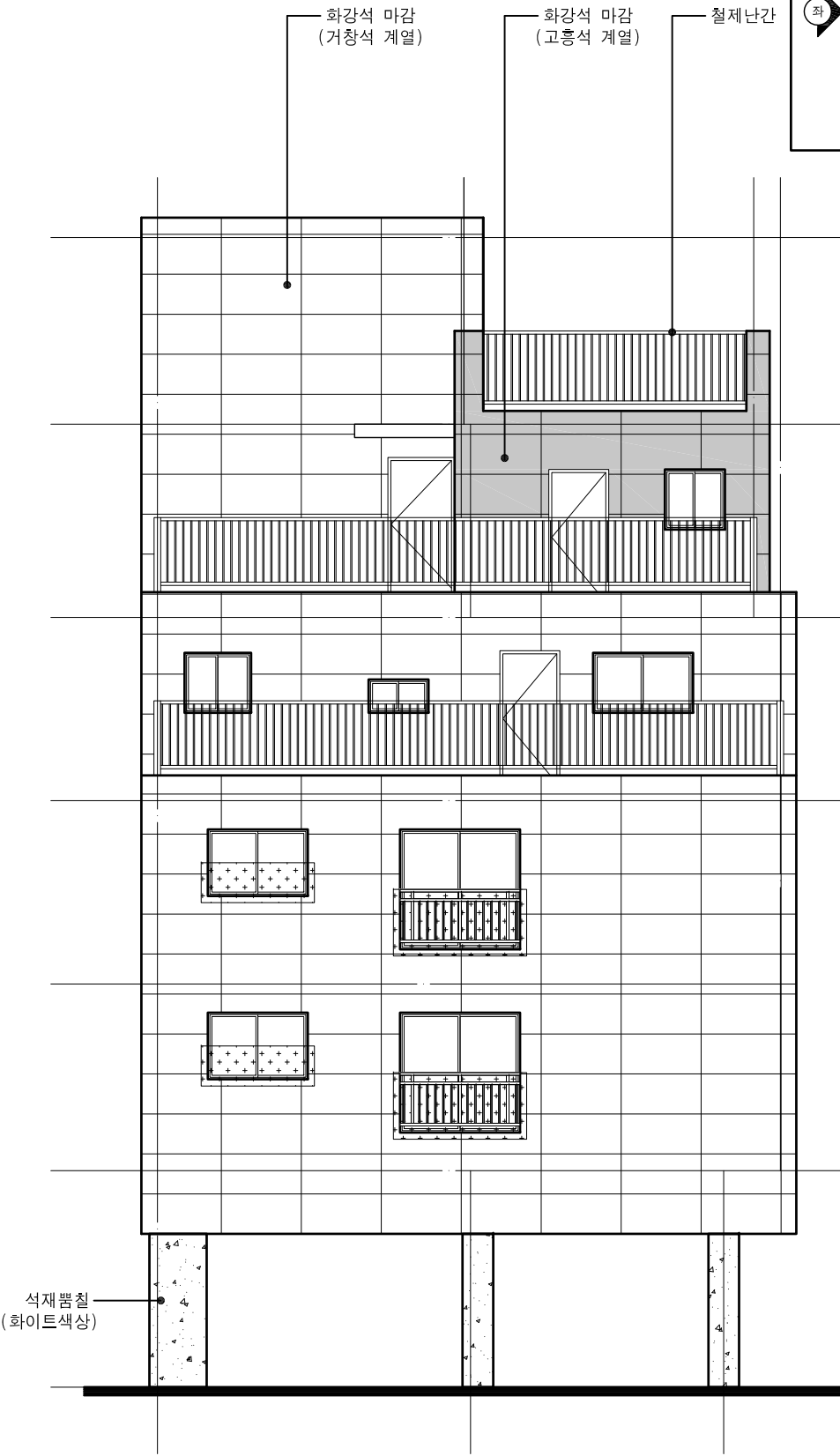
배 면 도 SCALE : A3 : 1/100
